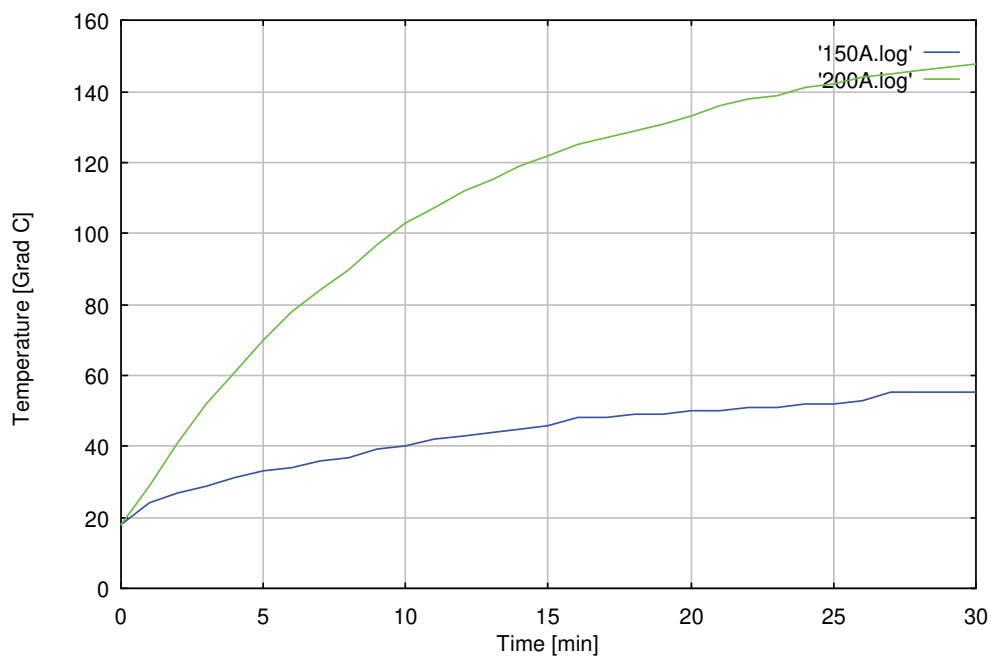
Abb. 5: Erwärmungskurven bei Dauerstrombelastung. Fig. 5: Heat-Up Characteristics at continuous current.
